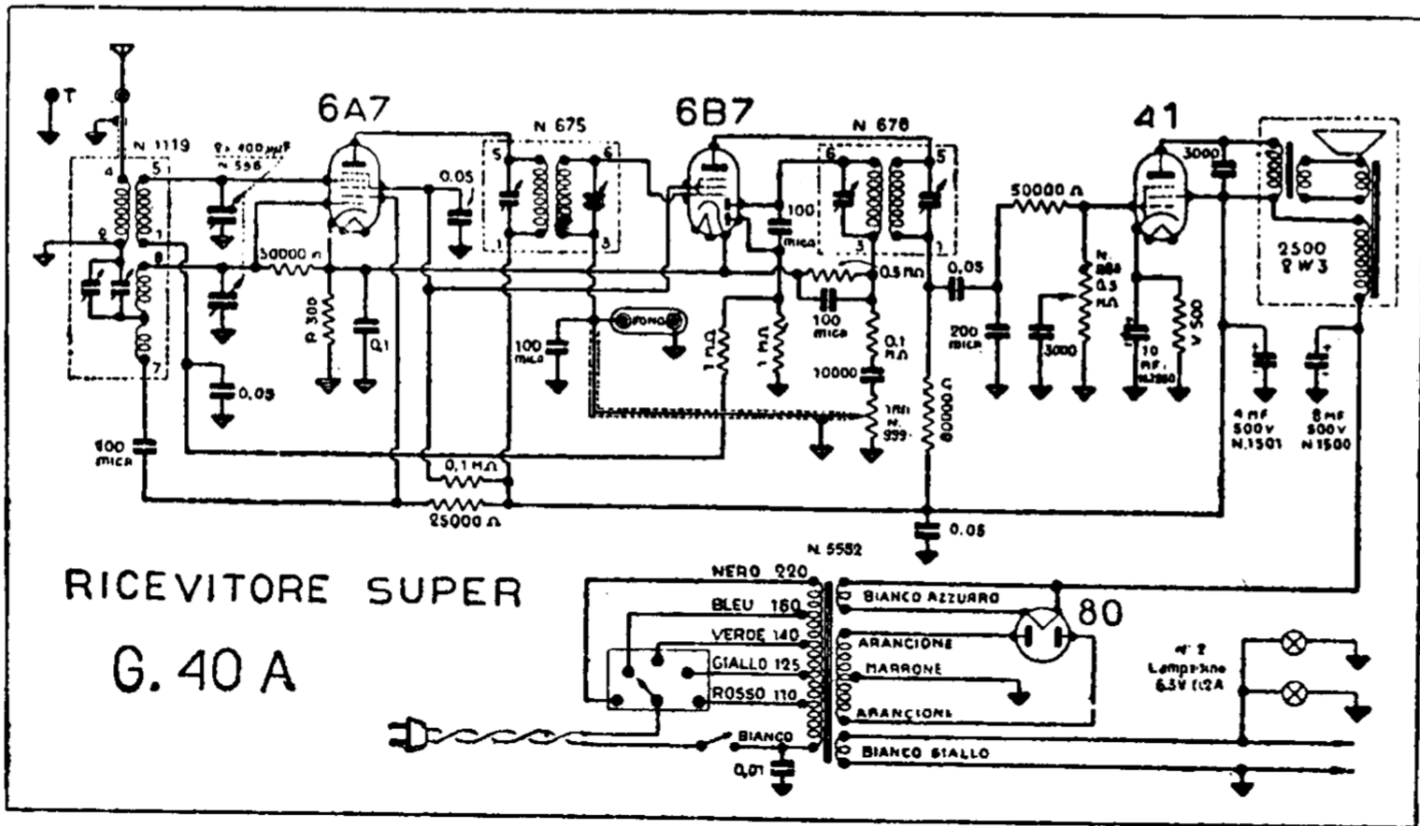
S. A. GELOSO. — Mod. G. 40 A. — Super a circuito riflesso. — Media frequenza: 467 kHz. Produzione 1937.
